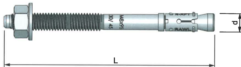
Rysunek A1. Łącznik rozporowy R-XPT
